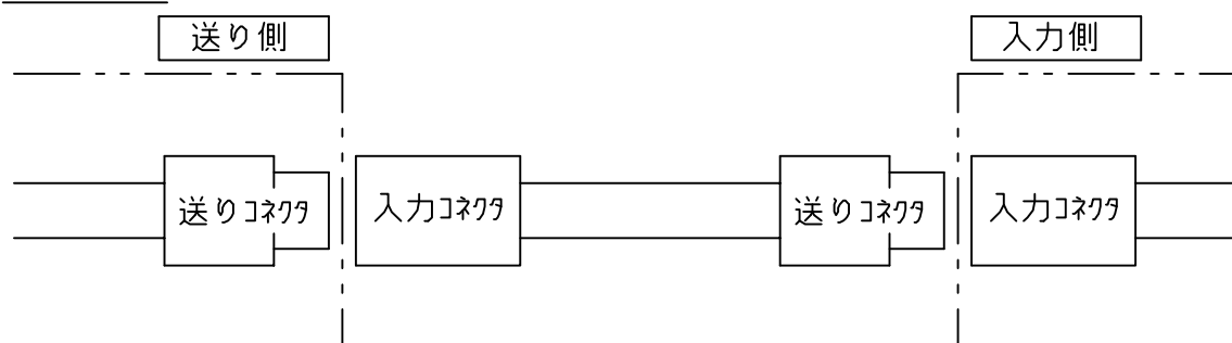
電気接続図
