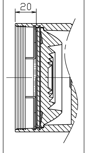
装着時寸法
