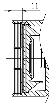
装着時寸法
