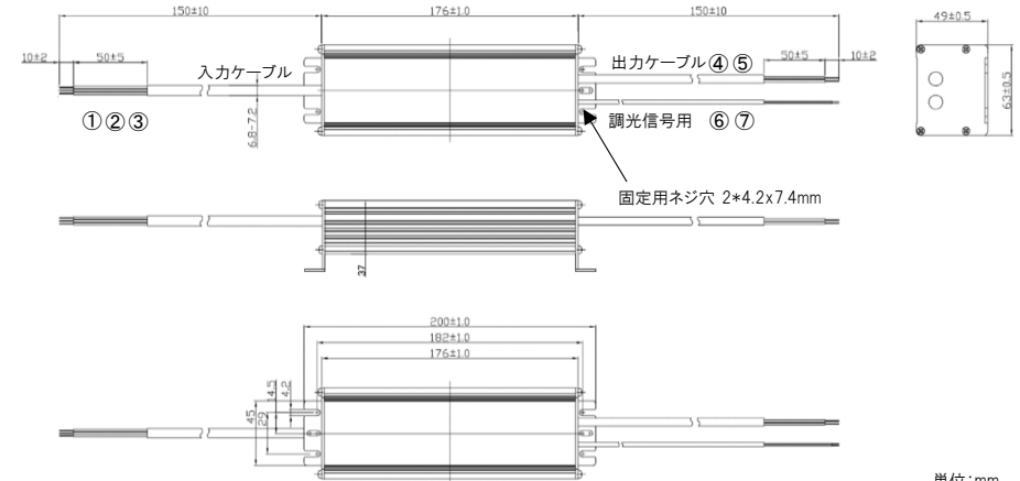
単位:mm
