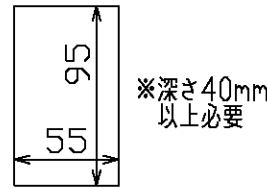
ボックス取付け埋込寸法 (S=1/4)
