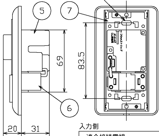
ボックス取付け埋込寸法 (S=1/4)
