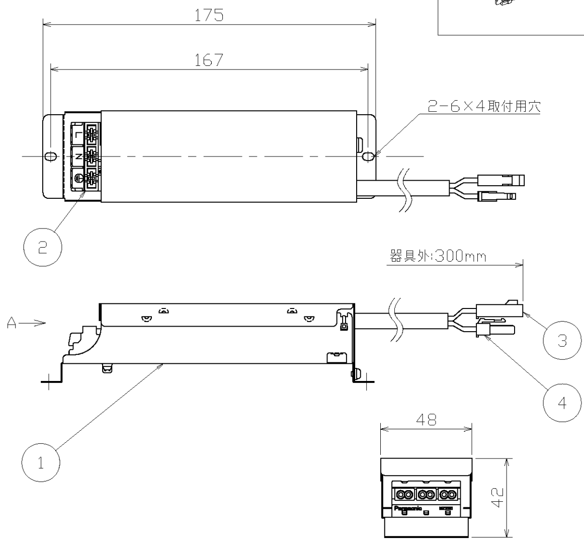
A矢視図
