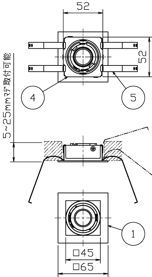
指定灯具取付状態図
